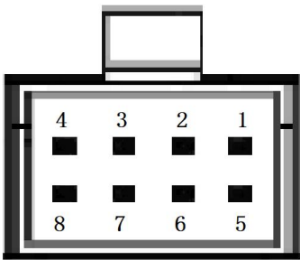
图 3.针脚示意图
