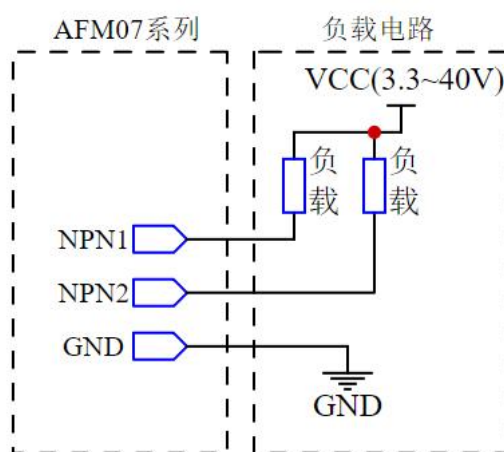
图 10.NPN 控制上下限原理图
