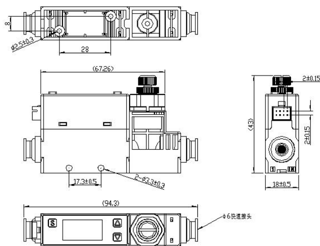
图 5.AFM08 系列针阀尺寸图（单位：mm；未注明公差：±0.5mm）
