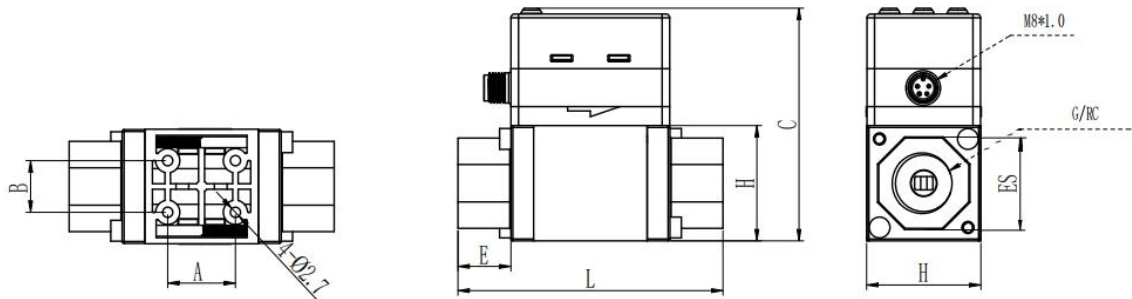
图8. JDL9025系列外形尺寸图（单位：mm，L公差：±1mm,其余未标公差：±0.5 mm）
