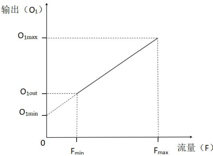
图 4. JDL9000系列流量与输出的对应线性图
