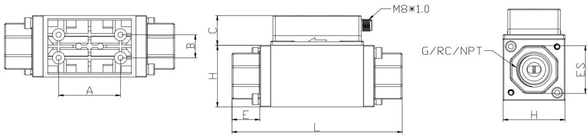
图8. JDL9010系列外形尺寸图（单位：mm，L公差：±1mm,其余未标公差：±0.5mm）
