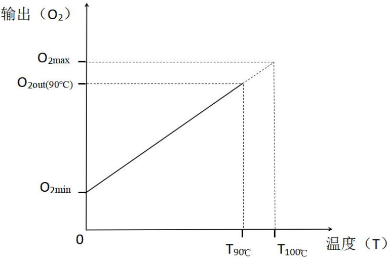
图 7. JDL9000系列温度与输出的对应线性图
