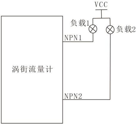
图 5. NPN 输出典型电路图
